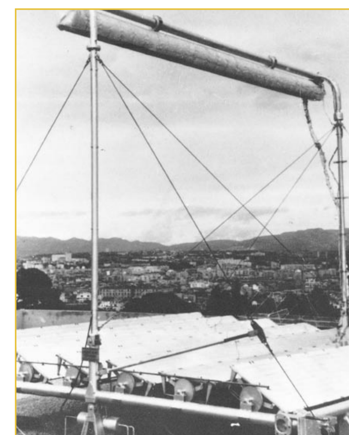
Fig. 6 - Il primo impianto solare a concentrazione lineare a specchi piani o di tipo Fresnel progettato da Giovanni Francia a Genova e installato a Marsiglia con la collaborazione di Marcel Perrot nel 1964 (Fotografia per cortesia degli eredi di Francia).
