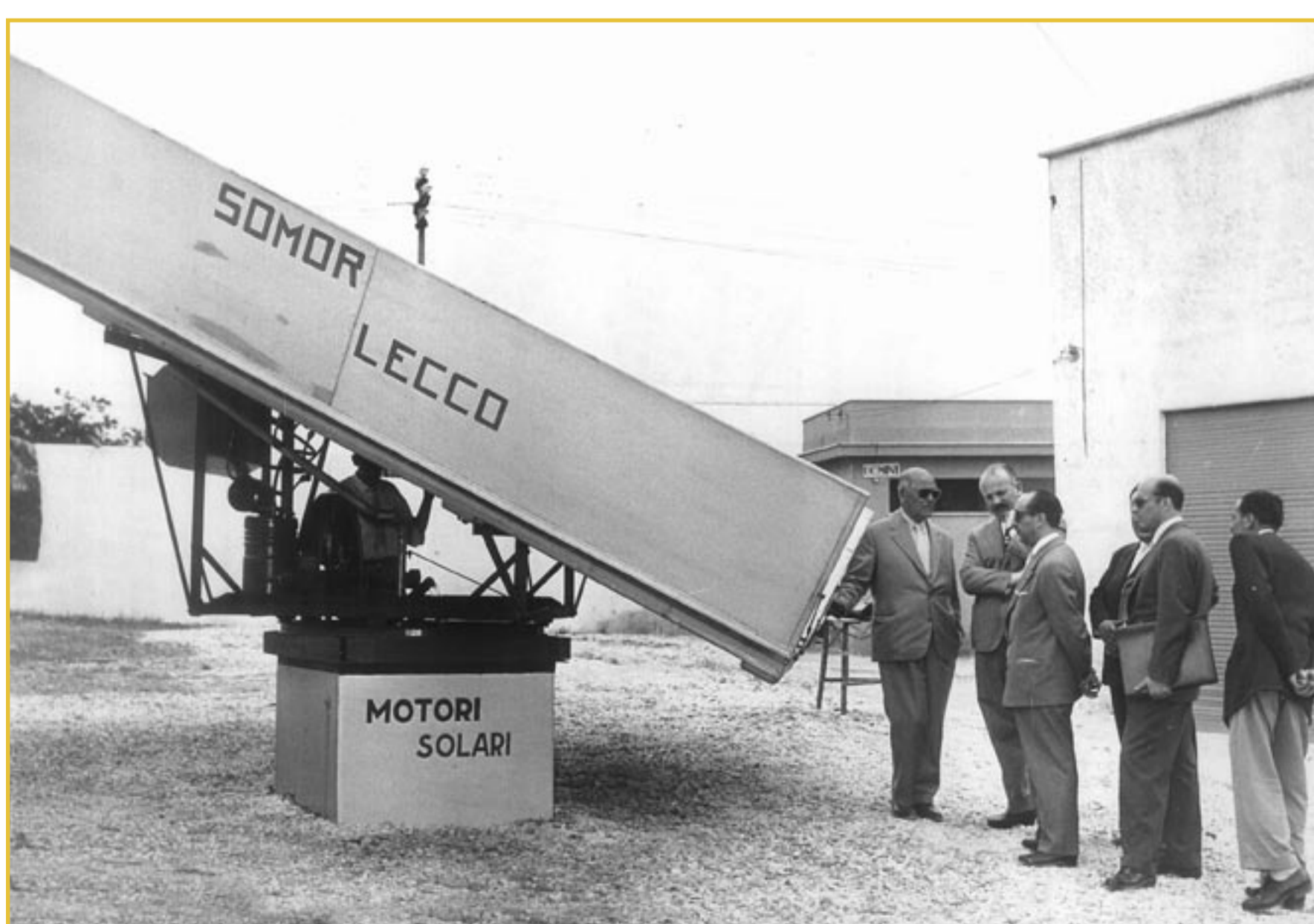
Fig. 2 - La pompa solare Somor, inventata nel 1948 e brevettata nel 1951 da Ferruccio Grassi di Lecco. La pompa Somor fu esposta in occasione del primo Congresso mondiale sull'energia solare tenuto nel 1955 in Arizona (Stati Uniti) nella città di Phoenix, organizzato dall'AFASE (Association for Applied Solar Energy), dalla quale ebbe origine l'attuale International Solar Energy Society (ISES) (Fotografia per cortesia degli eredi di Grassi).
